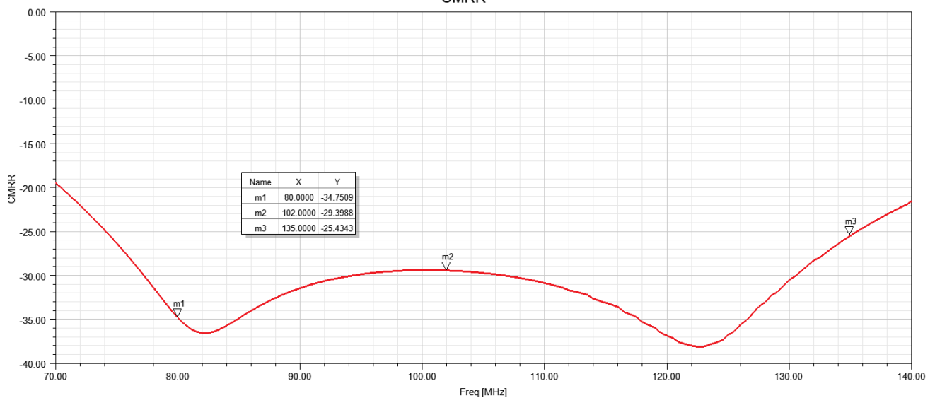
CMRR
