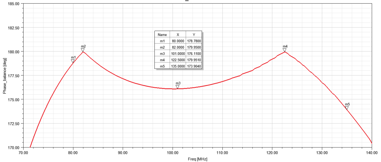
Amplitude_Balance
