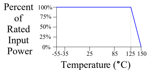
额定功率温度特性曲线
